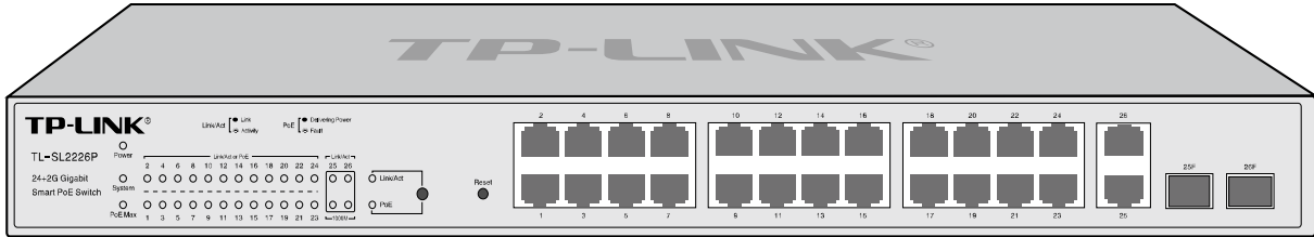
图 2-2 TL-SL2226P 前面板
